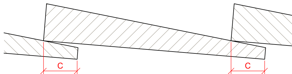
Samledetalje / Verbindungsdetail
