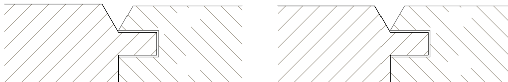
Samledetalje / Verbindungsdetail / assembly detail
