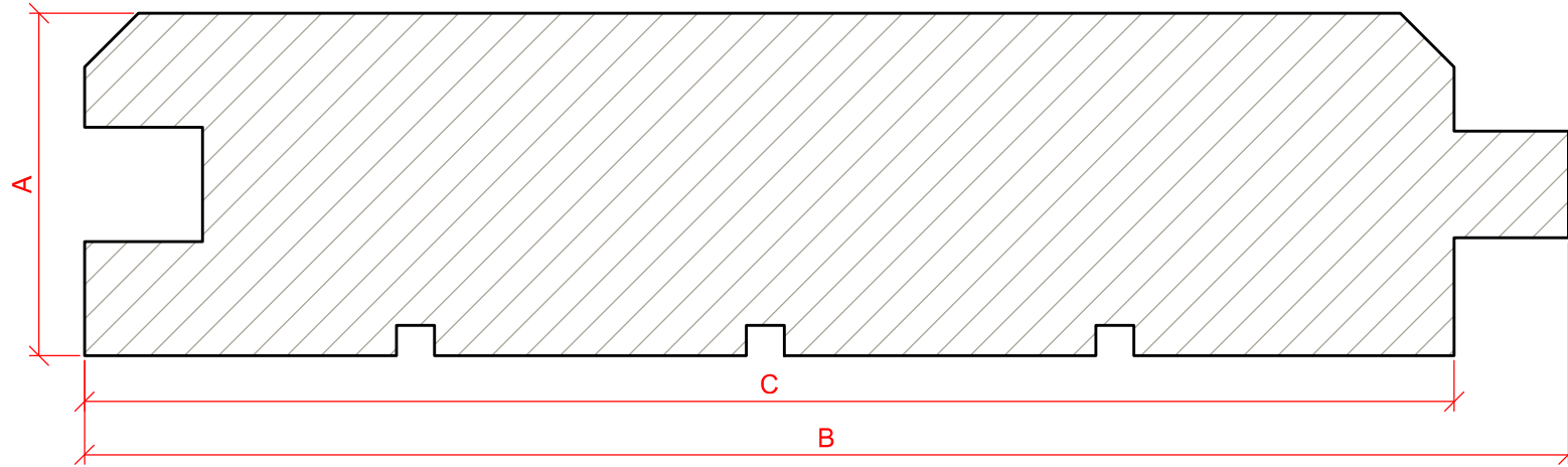
Samledetalje / Verbindungsdetail
