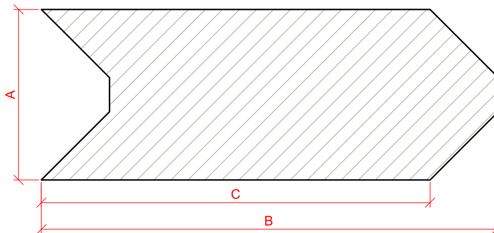
Samledetalje / Verbindungsdetail
