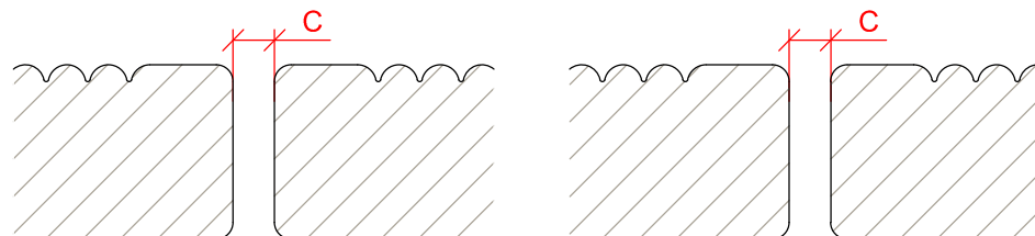
Samledetalje / Verbindungsdetail
